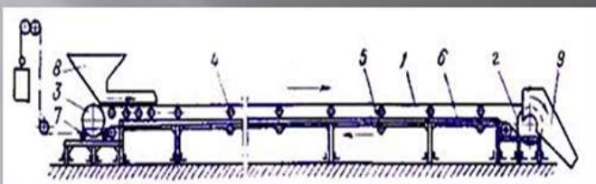
Схема стрічкового конвеєра: 1 – стрічка; 2 – приводний барабан; 3 – натяжний барабан; 4 – роликіві опори; 5 – роликіві опори порожньої гілки; 6 – опірня рама; 7 – натяжний пристрій; 8 – завантажувальня лійка; 9 – розвантажувальний жолоб
